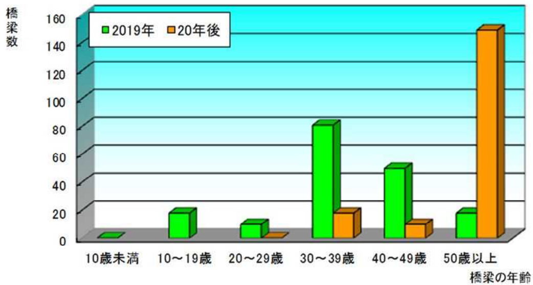
高齢化橋梁の分布の変化
